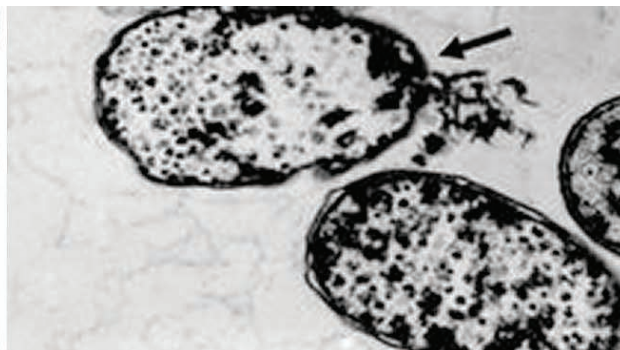
Pohľad na odolné bunky E. coli vystavené účinkom polyméru PHMG
