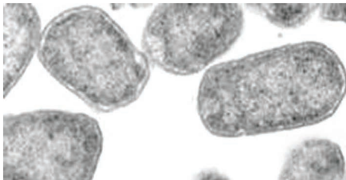
Pohľad na odolné bunky E. coli vystavené účinkom polyméru PHMG
